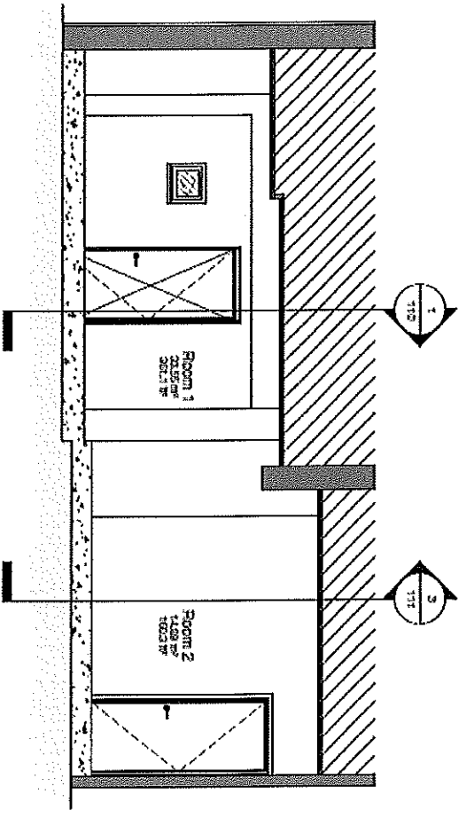
Section 3 1 : 50 0/43
